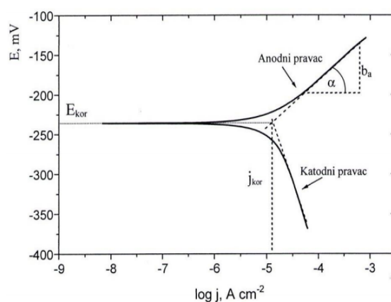
Slika 11. Princip Tafelove ekstrapolacije 4
