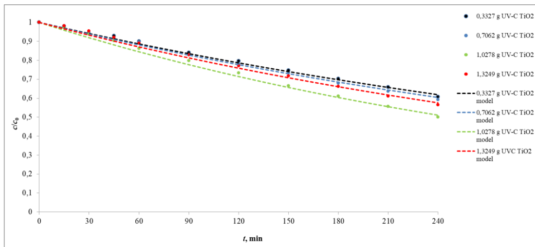
Slika 4.6. Utjecaj mase fotokatalitičkog sloja na fotokatalitičku razgradnju imidakloprida uz primjenu Arcadia natural sunlight lampe ( c_{10}=10 mg/L, Q_R=1,4 L/min, m(\text{TiO}_2)=0,3327-1,3249 g)
