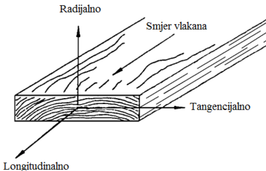
Slika 1. Ortotropija drva 1
