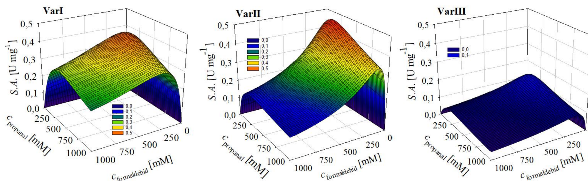
Slika 4.6. Utjecaj koncentracije formaldehida i propanala na specifičnu aktivnost enzima FSA VarI/VarII/VarIII u reakciji aldolne adicije (25 °C, 50 mM pufer, \gamma_{\text{FSA}} = 0,5 \text{ mg mL}^{-1} )
