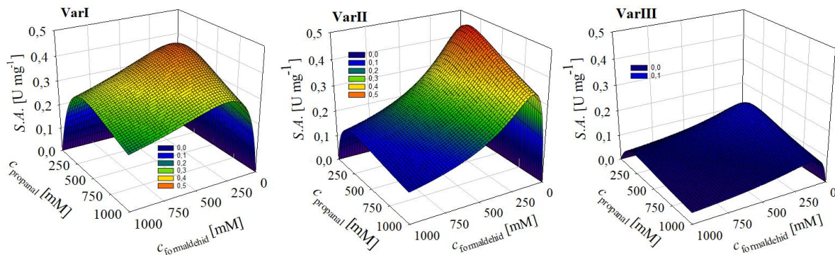
Slika 4.6. Utjecaj koncentracije formaldehida i propanala na specifičnu aktivnost enzima FSA VarI/VarII/VarIII u reakciji aldolne adicije ( 25\text{ }^{\circ}\text{C} , 50\text{ mM} pufer, \gamma_{\text{FSA}} = 0,5\text{ mg mL}^{-1} )
