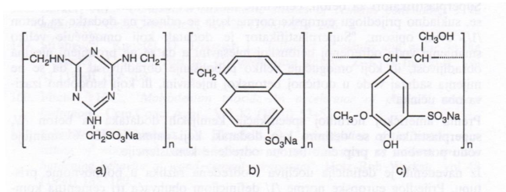
Slika 2.7. Reprezentativni segmenti polimera iz kemijskog sastava superplastifikatora: a) sulfonirani melamin-formaldehidni kondenzati (SMF), b) sulfonirani naftalen-formaldehidni kondenzati (SNF), c) modificirani lignosulfonati (MLS)
