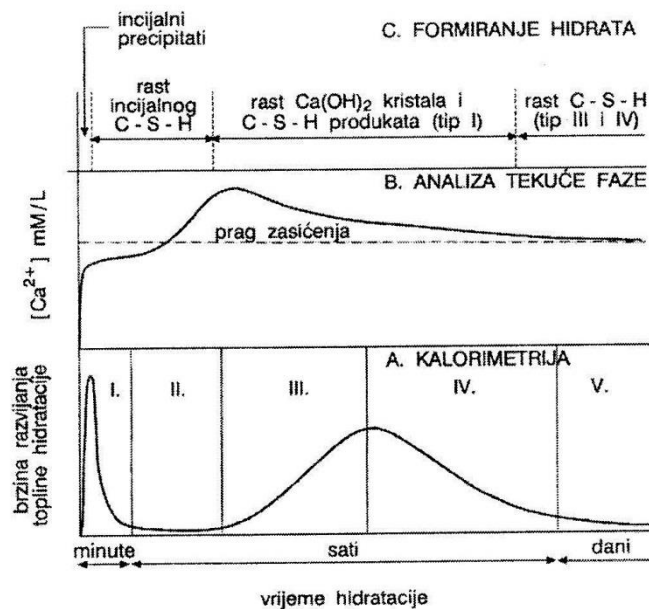
Slika 2.2. Shematski prikaz promjena u sustavu C_3S -voda (omjer voda-čvrsto < 1 ) u tijeku napredovanja hidratacije
