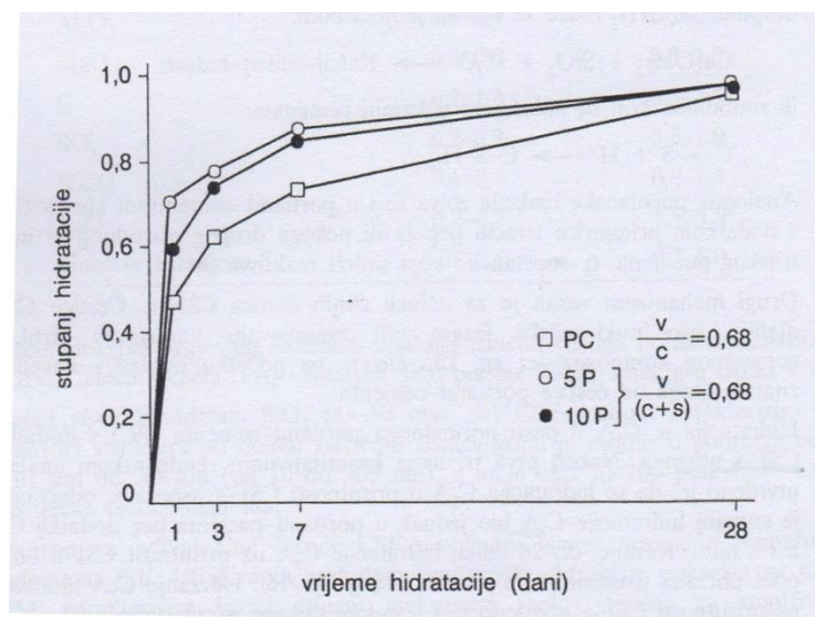
Slika 2.10. Stupanj hidratacije alita u funkciji vremena hidratacije u portland-cementni pastama s dodatkom 0 % (PC), 5 % (5P) i 10 % (10P) CSF-a koje su imale omjer između vode i veziva 0,68 15
