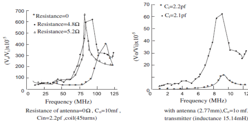
Slika 6.8. Grafički prikaz ovisnosti otpora i frekvencije s obzirom na omjer V_{out} / V_{in}
