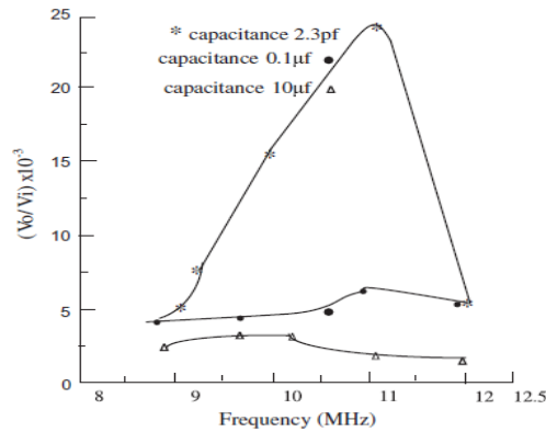
Slika 6.7. Grafički prikaz ovisnosti kapaciteta i frekvencije s obzirom na omjer V_{out} / V_{in}
