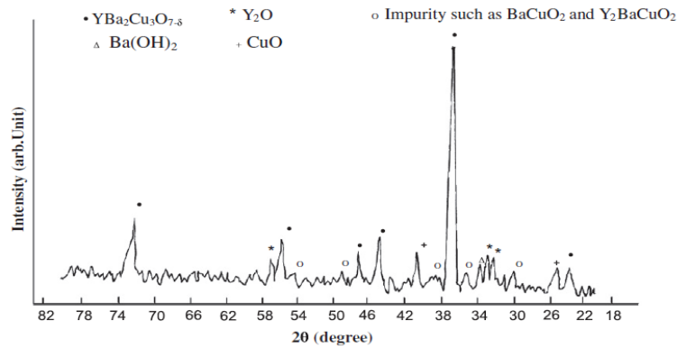
Slika 6.8. Prikaz rendgenske difrakcije uzorka konačnog praha \text{YBa}_2\text{Cu}_3\text{O}_{7-\delta}
