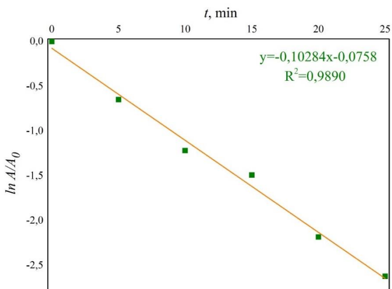
Slika 42. Kinetika razgradnje HCQ-a, LED 365 nm, 0,10 mg TiO 2 /mL
