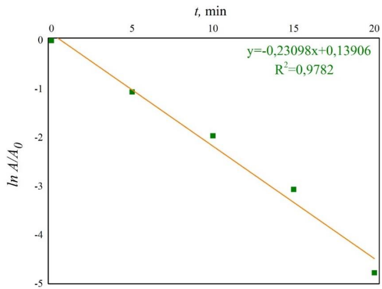
Slika 43. Kinetika razgradnje HCQ, LED 365 nm, 0,5 mg TiO 2 /mL
