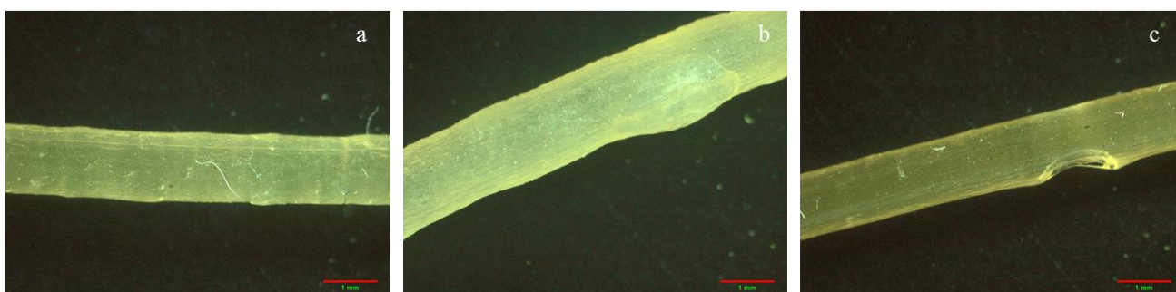
Slika 24. Mikrografije filamenata: a) PVA FF 10% 150, b) PVA FF 10% 160, c) PVA FF 10% 170 pri uvećanju 1,25x
