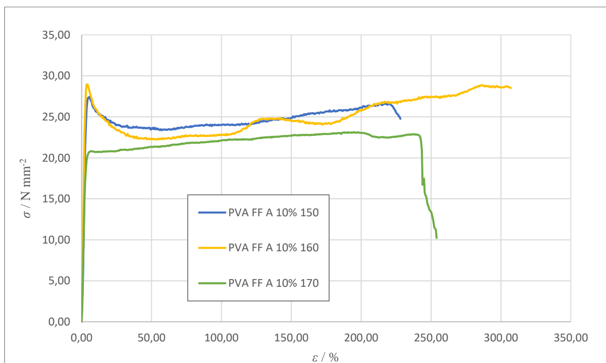
Slika 28. Dijagram napreznja za uzorke filameta PVA Formfutura Atlas
