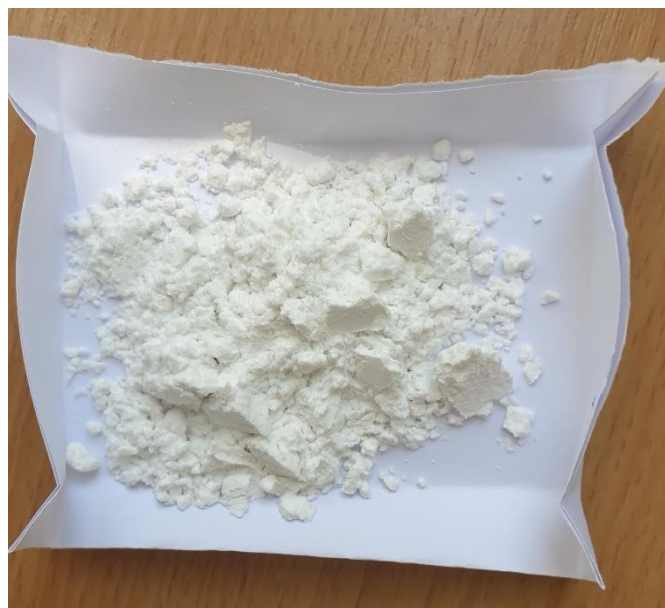
Slika 11. Dronedaron-hidroklorid
