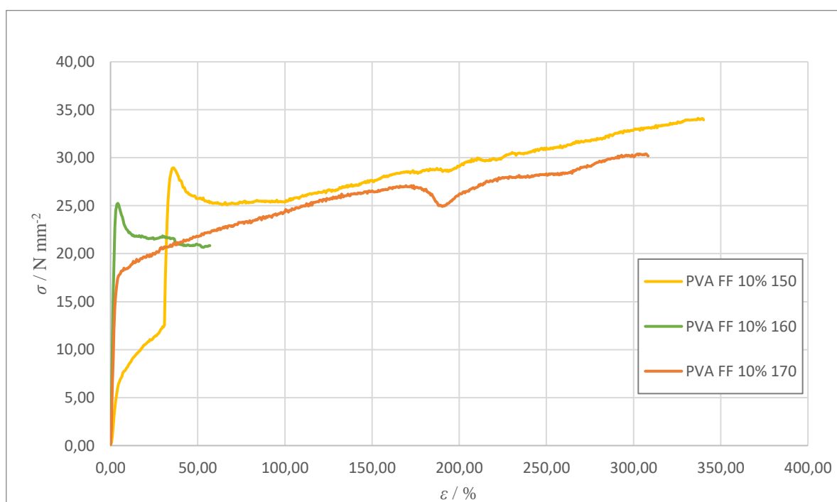
Slika 30. Dijagram napreznosti za uzorke filameta PVA Aqua Solve
