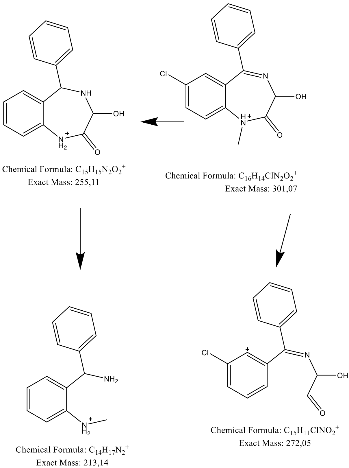
Slika 23. Predložena fragmentacija DP-2
