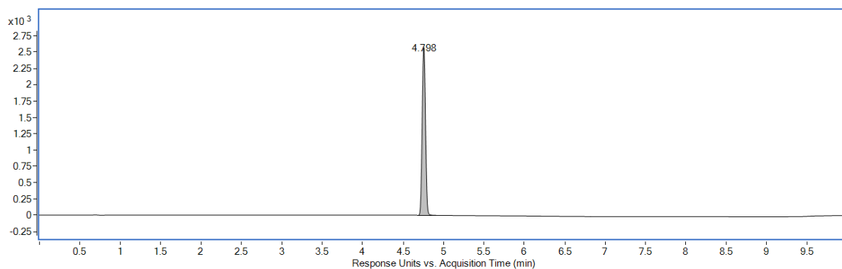
Slika 11. Kromatogram ne tretiranog diazepama (konc. 1 mg/mL)
