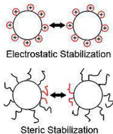
Slika 6. Grafički prikaz elektrostatske i prostorne stabilizacije [2].
