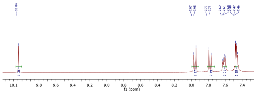
Slika 1. ^1\text{H} -NMR spektar spoja 1
