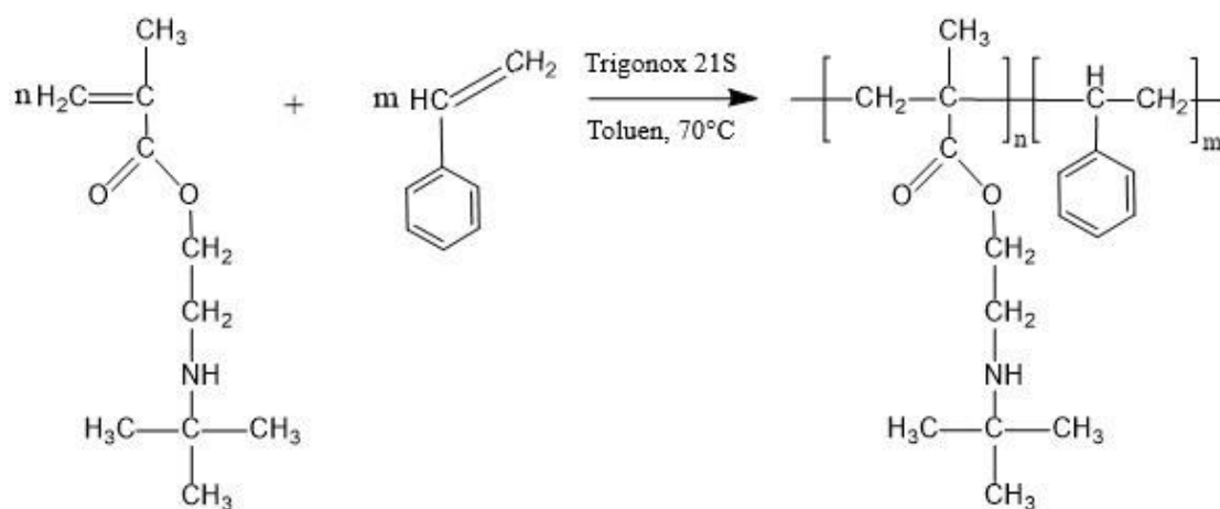
Slika 16. Shema radikalске kopolimerizacije TBAEMA i: a) MMA b) ST i c) ODMA.
