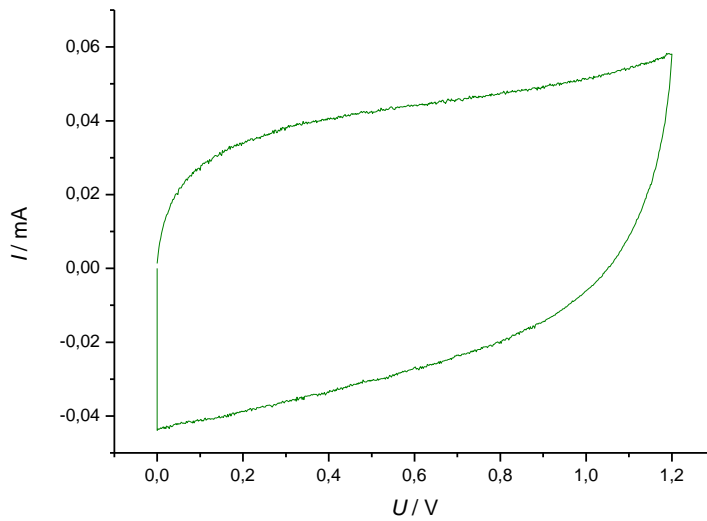
Slika 4.9. Ciklički voltamogram za Superkondenzator2 , u 0,5 \text{ mol dm}^{-3} \text{ Na}_2\text{SO}_4 , pri v = 50 \text{ mV s}^{-1}
