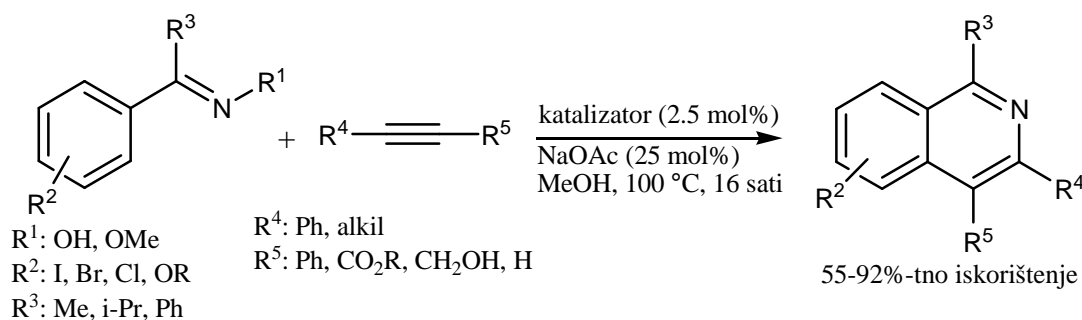
Shema 10. Sintaza supstituiranih izokinolina rutenijem kataliziranom reakcijom ciklizacije ketoksima i alkinima
