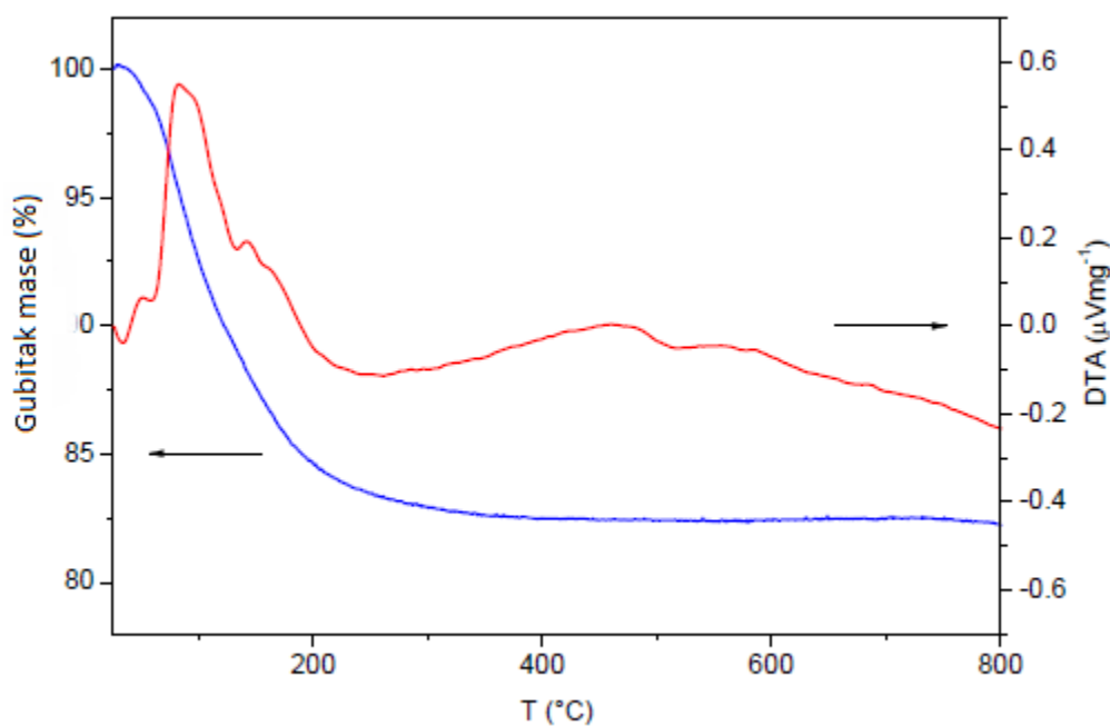
Slika 7. DTA i TGA krivulje pripremljenih titanatnih nanocjevčica dobivene zagrijavanjem od 10\text{ }^{\circ}\text{C min}^{-1} u zraku.
