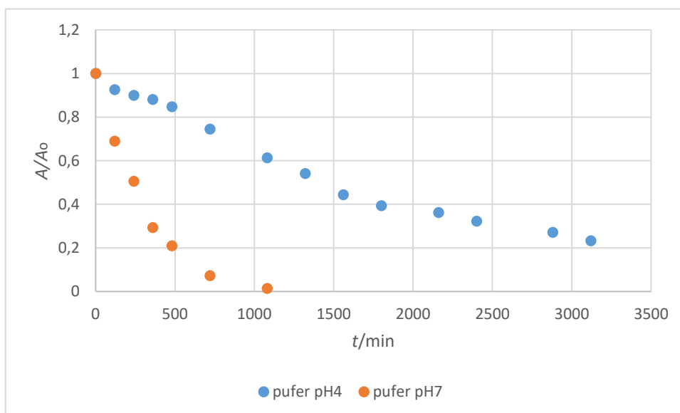
Slika 28. Razgradnja hidroksiklorokina u puferskim otopinama pH-vrijednosti 4 i 7
