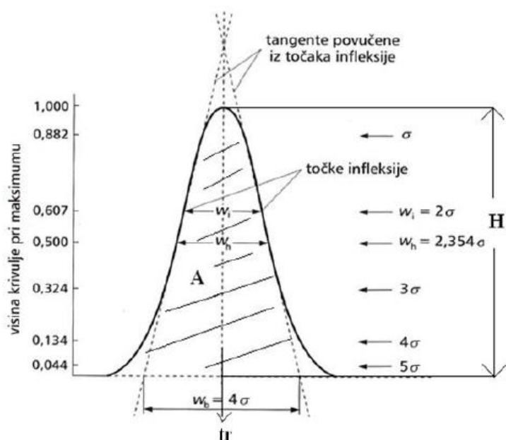
Slika 6. Karakteristična svojstva kromatografske krivulje [16]
