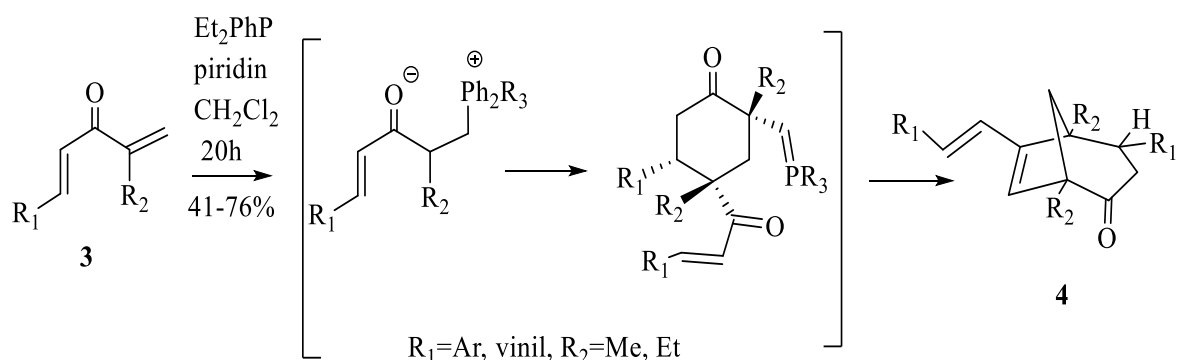
Shema 2. Fosfinska dimerizacija 1,4-diena-3-ona.
