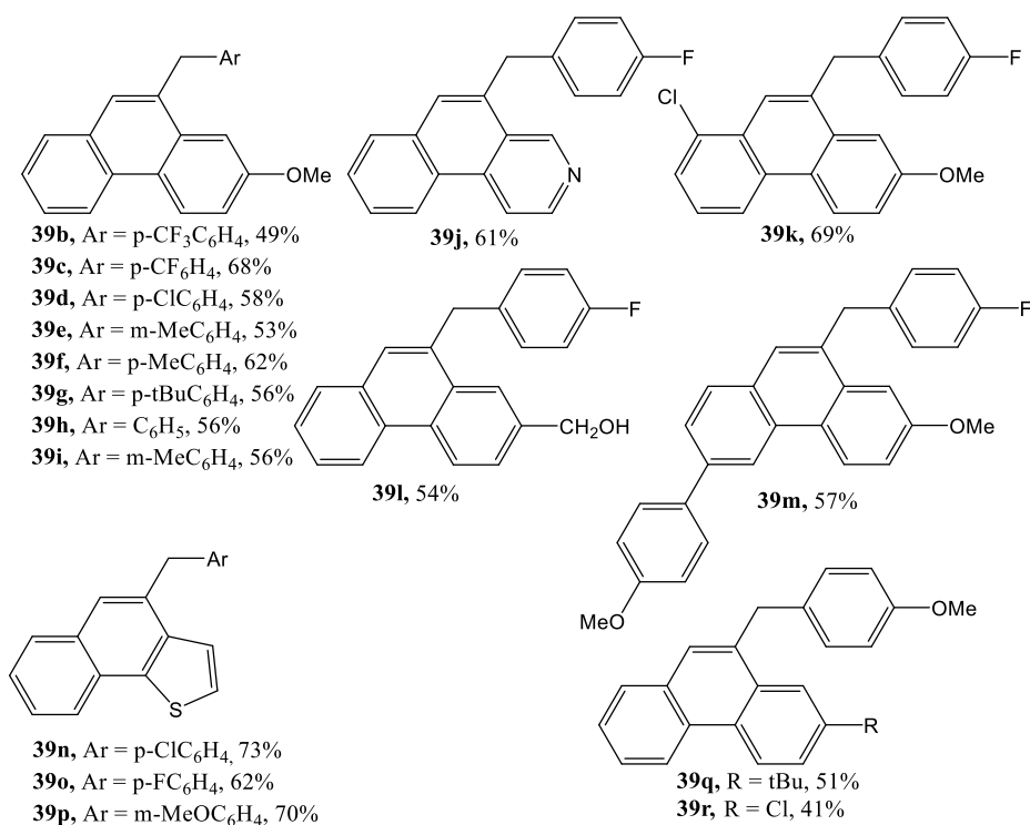
Shema 17. Sintaza derivata fenantrena 39b-r
