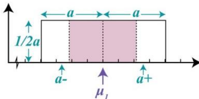
Slika 7: Pravokutna raspodjela 20
