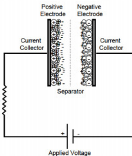
Slika 2.14. Shema superkondenzatora [23]
