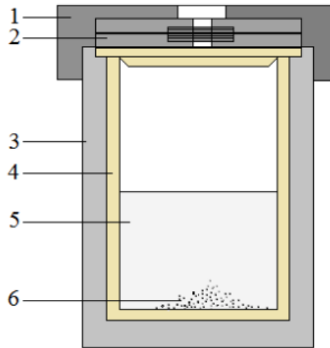
Slika 2.6. Shematski prikaz hidrotermalnog autoklava (1-poklopac od nehrđajućeg čelika, 2-potisni disk, 3-posuda od nehrđajućeg čelika, 4-teflonska posuda s teflonskim poklopcem, 5-otapalo, 6-reagens)
