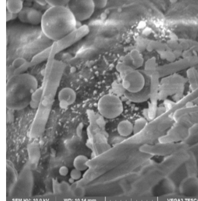
Slika 4.3 SEM mikrografi letečeg pepela (FA/T3P) modificiran s TEOS i PEGom, kod različitih povečana
