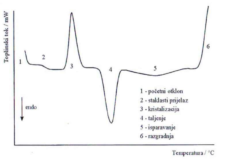
Slika 14. DSC termogram 2
