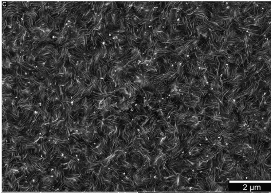
Slika 7. SEM prikaz kompozita LDPE/3wt % ZnO 13
