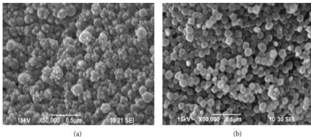
Slika 17. SEM prikaz nanočestica silicijevog dioksida koji sadržava imobilizirane nanočestice srebra (a) i bakra (b) 10
