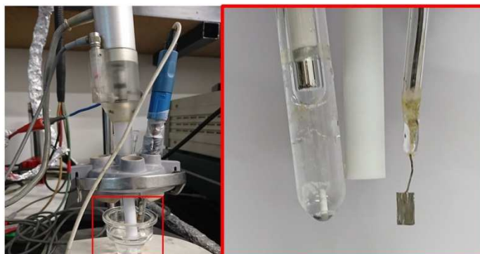
Slika 3.3. Čelija i troelektrodni sustav za elektrokemijsku sintezu sloja PEDOT i kompozita PEDOT/grafen
