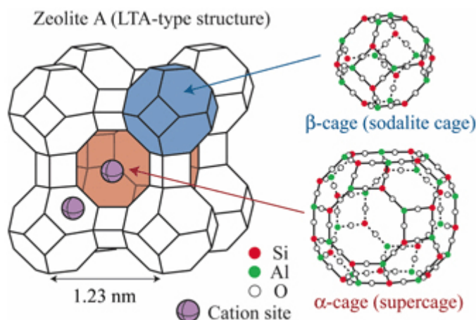
Slika 3.4. Struktura zeolita [29]
