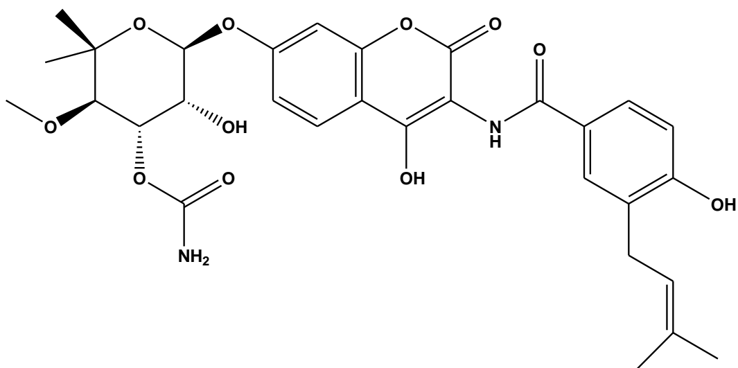
Slika 10. Novobiocin
