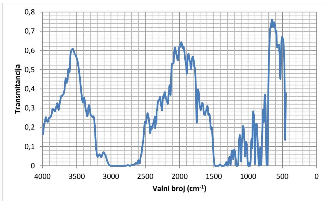
Slika 93. Transmisijski spektar PP folije debljine 500 μm.
