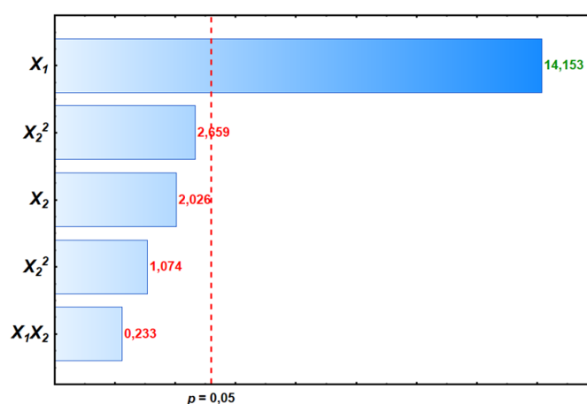
Slika 6. Pareto prikaz utjecaja pojedinih parametara u modelu fotokatalitičke razgradnje memantina.
