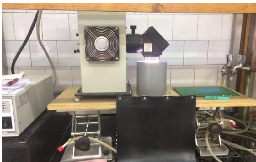
Slika 3.3. Simulator sunčeva zračenja
