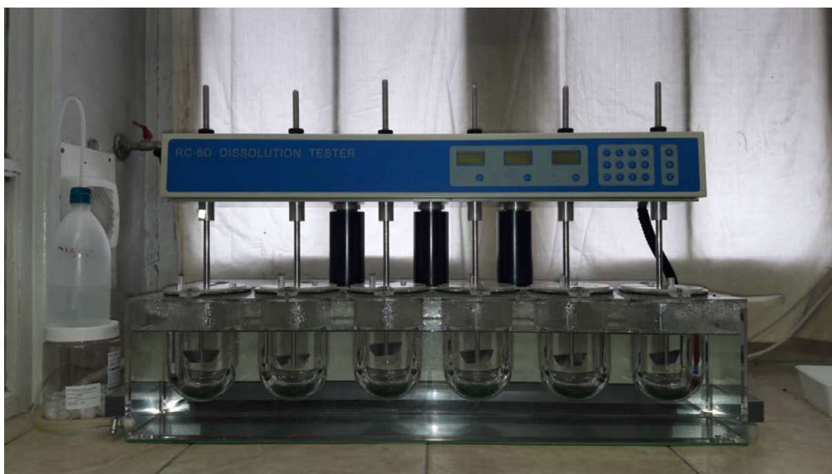
Slika 3.6. Fotografija uređaja za određivanje profila otpuštanja djelatne tvari RC-6D (Zhengzhou Nanbei Instruments, Zhengzhou, NR Kina).
