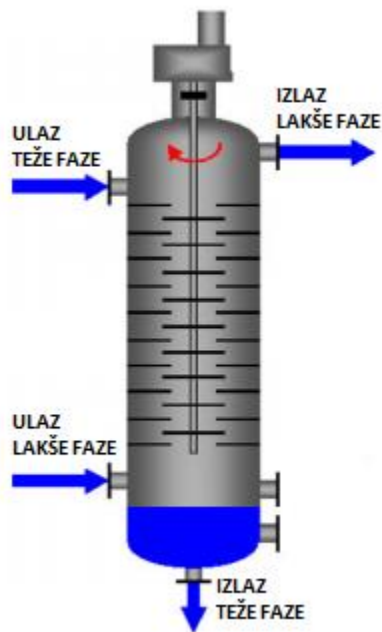
Slika 3. Ekstrakcijska kolona [4]
