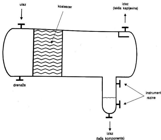
Slika 4. Vodoravni gravitacijski separator (dekanter) s koalescerom [2]
