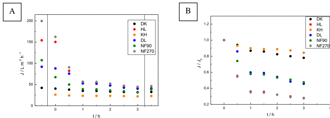
Slika 4.1. Ovisnost fluksa o vremenu za modelnu otopinu (A) i normaliziranog fluksa (B) za modelnu otopinu bez pesticida.
