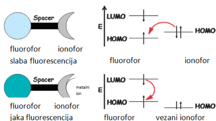
Slika 3. Fotoinducirani prijenos elektrona s prikazom molekularskih orbitala [6.]
