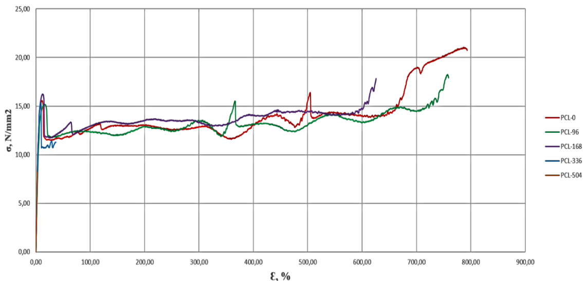
Slika 48. Krivulje naprezanje-istezanje za polikaprolakton (PCL) prije i nakon određenog vremena UV starenja
