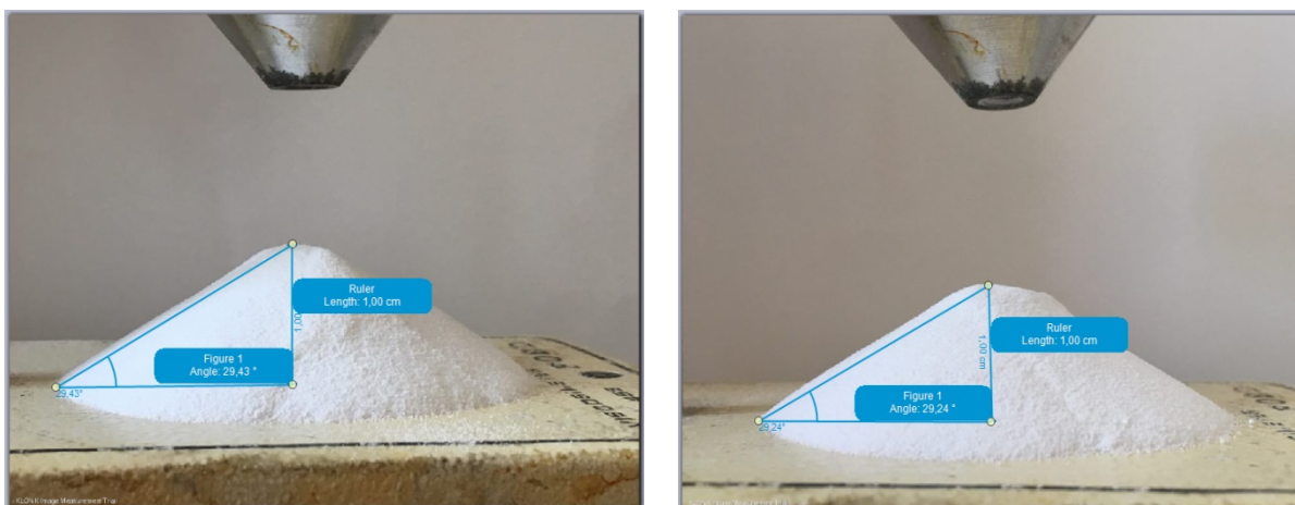
Slike 4.1. i 4.2. Fotografije formiranih stožaca za kolektive okrupnjenih jedinica G_LM+AZT_1 i G_LM+AZT_P; primjena KLONK Image Measurement softverskog paketa u određivanju kuta mirovanja.
