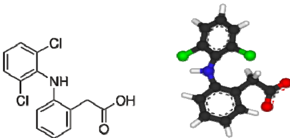
Slika 1. Prikaz strukture diklofenaka
