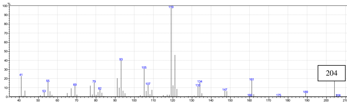
Slika 28. Prikaz masenog spektra italicena
