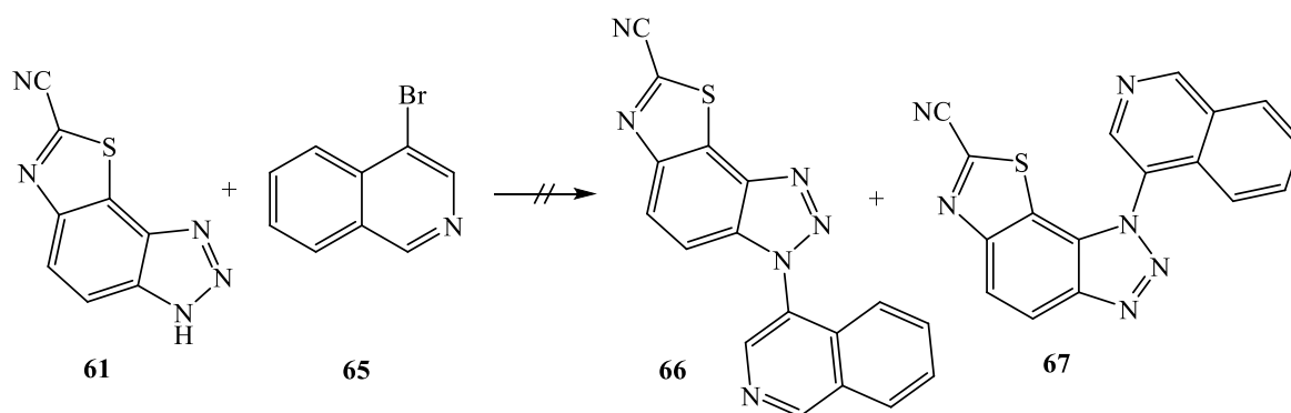
Shema 18. Kondenzacija tiazolobenzotriazola i 4-bromokinolina
