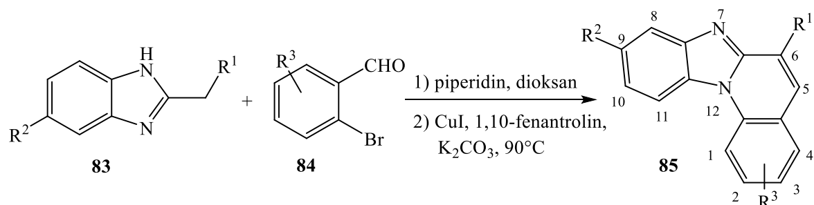
Tablica 5. Rezultati priprave supstituiranih benzimidazo[1,2- a ]kinolina
