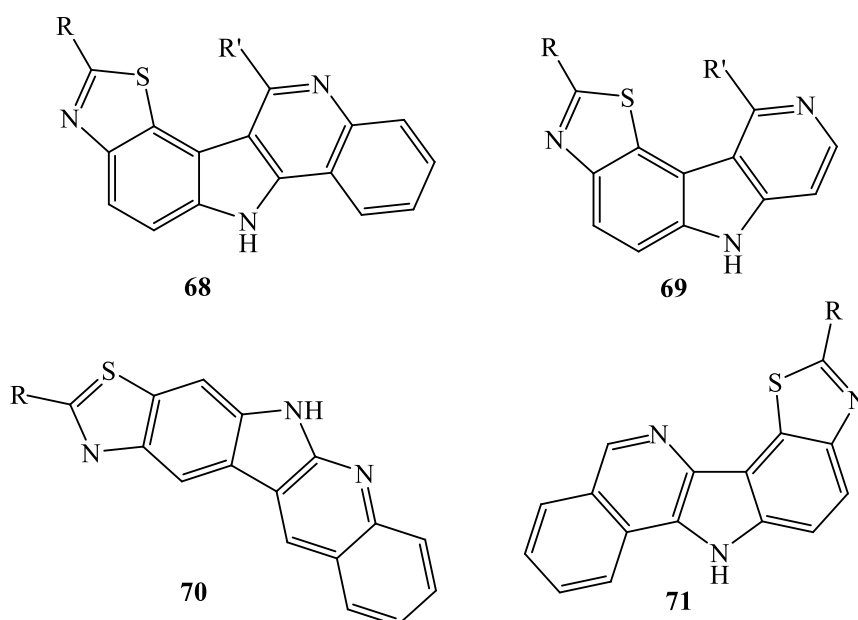
Slika 1. Strukture spojeva 68-71
