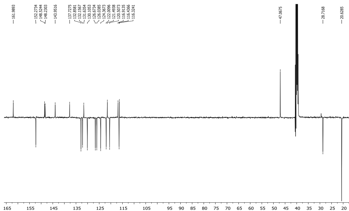
Slika 15. a) 1 H NMR spektar i b) 13 C NMR spektar N' -izobutilbenzo[ g ]benzo[4,5]imidazo[1,2- a ][1,5]naftiridin-7-karboksamida 15
