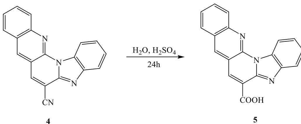
Shema 38. Priprava benzo[ g ]benzo[4,5]imidazo[1,2- a ][1,8]naftiridin-6-karboksilne kiseline 5
