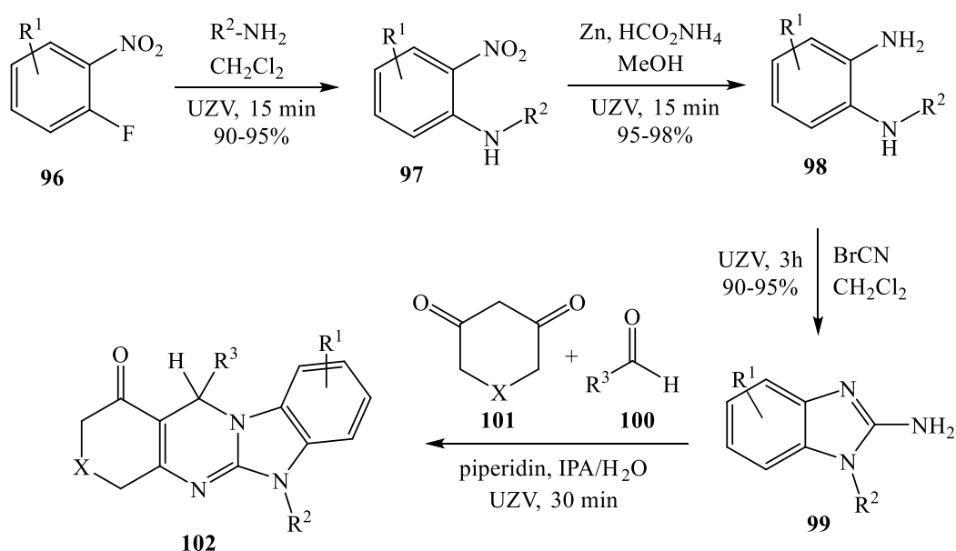
Shema 31. Ultrazvučna sinteza benzimidazo[2,1- b ]kinazolin-1(1 H )-ona
