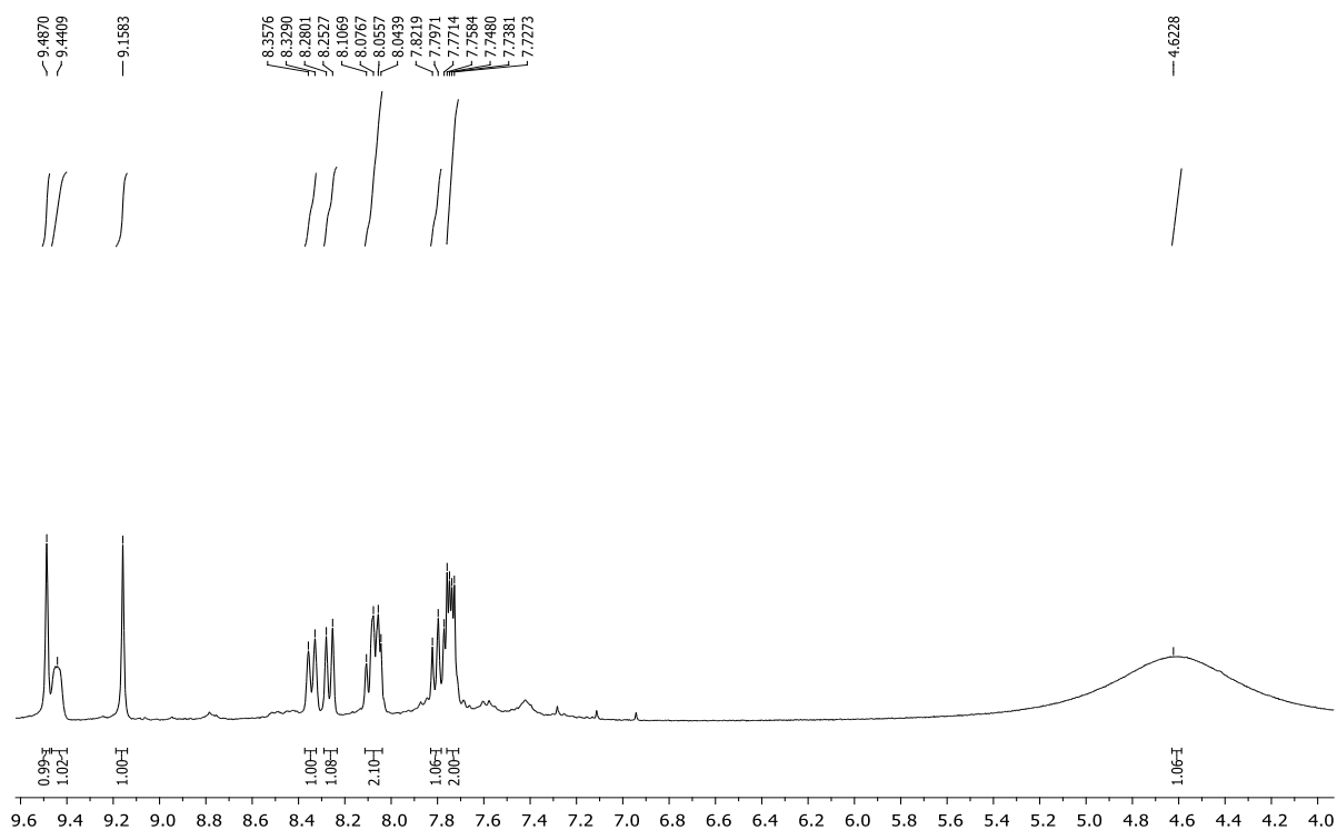
Slika 6. a) 1 H NMR spektar benzo[g]benzo[4,5]imidazo[1,2-a][1,8]naftiridin-6-karbonitrila 4 i b) 1 H NMR spektar benzo[g]benzo[4,5]imidazo[1,2-a][1,8]naftiridin-6-karboksilne kiseline 5
