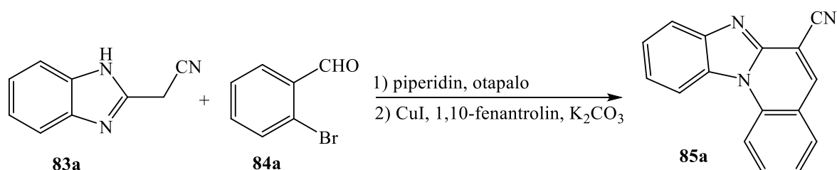
Shema 23. Sinteza cijano-supstituiranog benzimidazo[1,2- a ]kinolina
