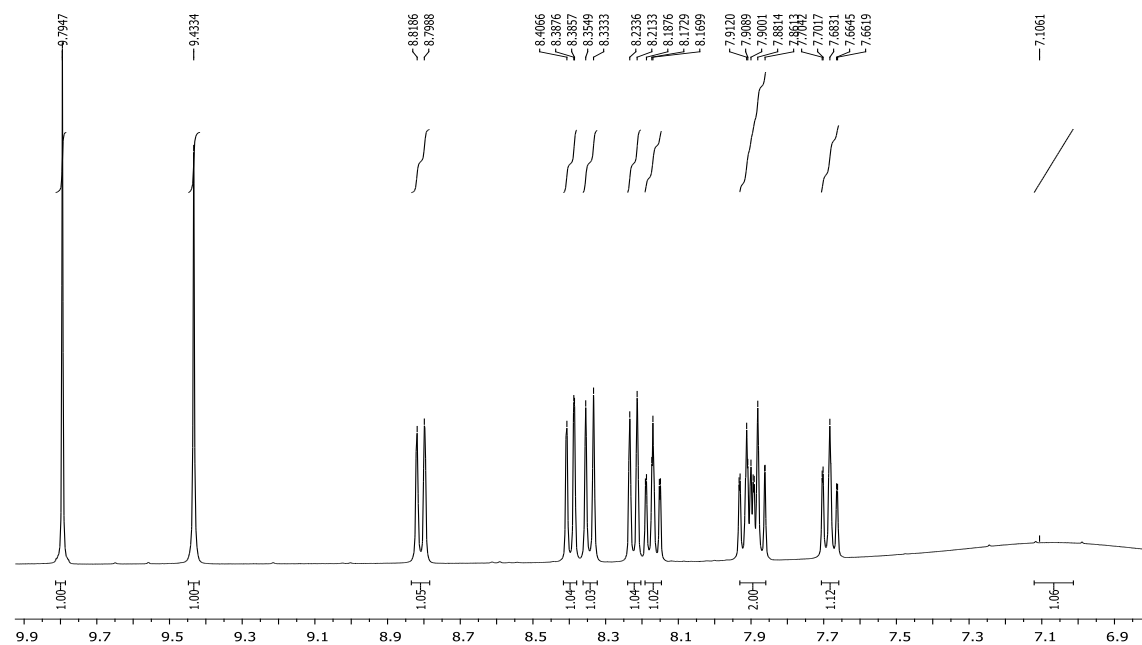
Slika 14. 1 H NMR spektar a) benzo[ g ]benzo[4,5]imidazo[1,2- a ][1,5]naftiridin-7-karbonitrila 12 i b) benzo[ g ]benzo[4,5]imidazo[1,2- a ][1,5]naftiridin-7-karboksilne kiseline
