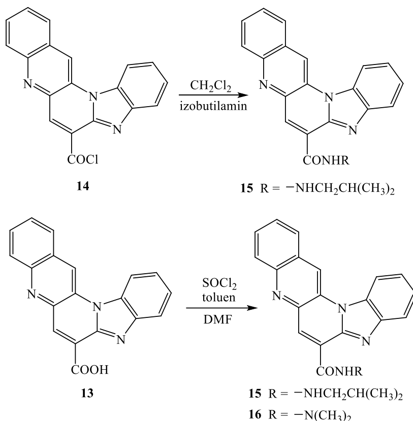
Shema 44. Priprava spojeva 15 i 16
