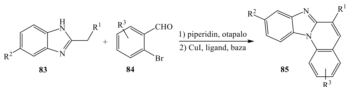
Shema 22. "One-pot" sinteza benzimidazo[1,2- a ]kinolina
