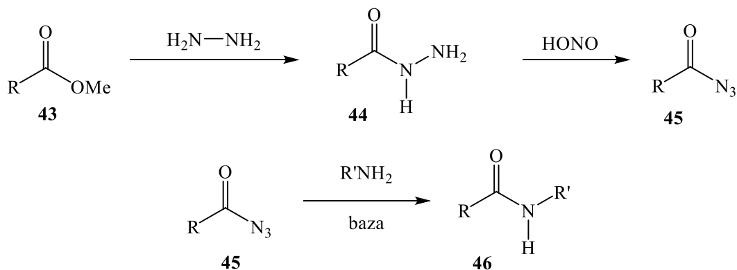
Shema 13. Sintaza amida preko generiranja acilnih azida
