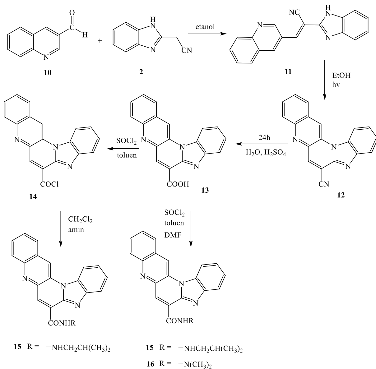
Shema 46. Sinteza derivata benzo[g]benzo[4,5]imidazo[1,2-a][1,5]naftiridina
