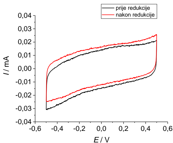
Slika 4.5. Ciklički voltamogram PEDOT sloja sintetiziranog iz otopine 0,01 \text{ mol dm}^{-3} PSS i 0,02 \text{ mol dm}^{-3} EDOT pri potencijalu 0,84 V tijekom 300 sekundi zabilježen prije i nakon polarizacije na potencijalu -1 V u trajanju od 300 sekundi
