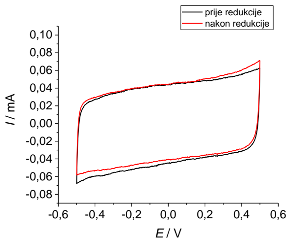
Slika 4.4. Ciklički voltamogram PEDOT sloja sintetiziranog iz otopine 0,01 \text{ mol dm}^{-3} PSS i 0,02 \text{ mol dm}^{-3} EDOT pri potencijalu 1,0 V tijekom 300 sekundi zabilježen prije i nakon polarizacije na potencijalu -1 V u trajanju od 300 sekundi
