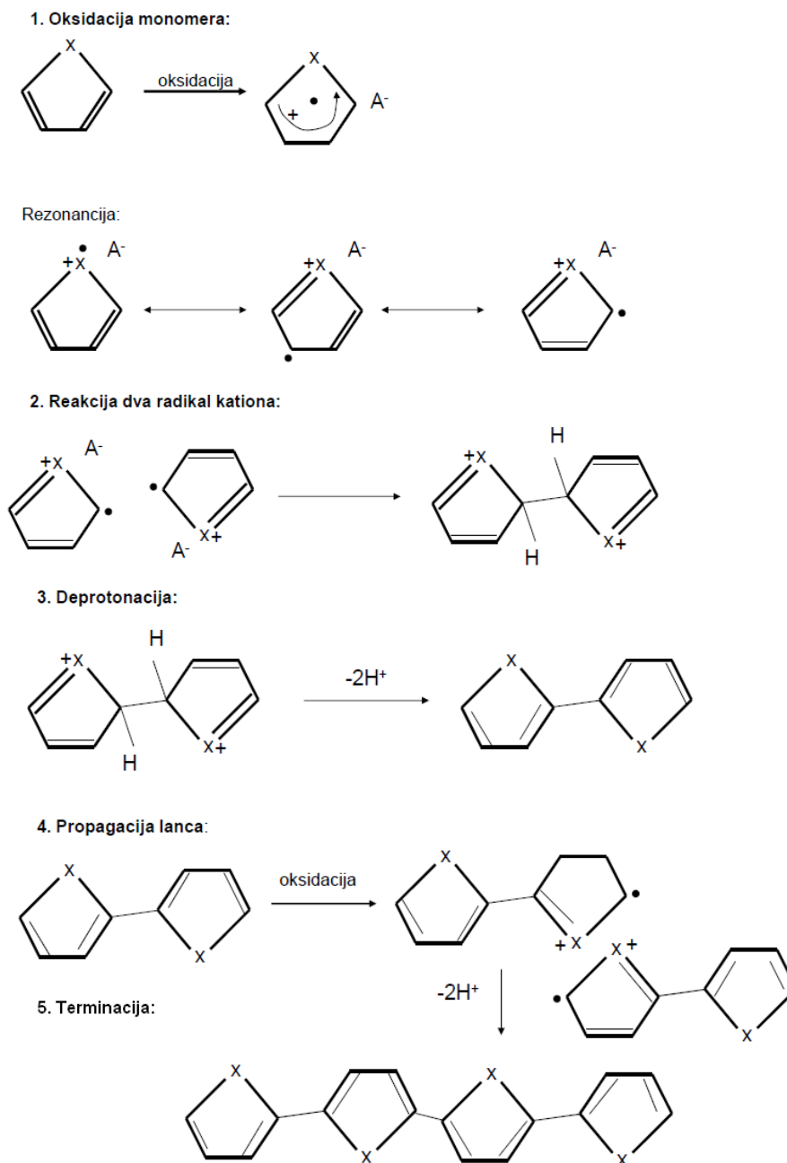
Slika 2.6. Shema polimerizacije
