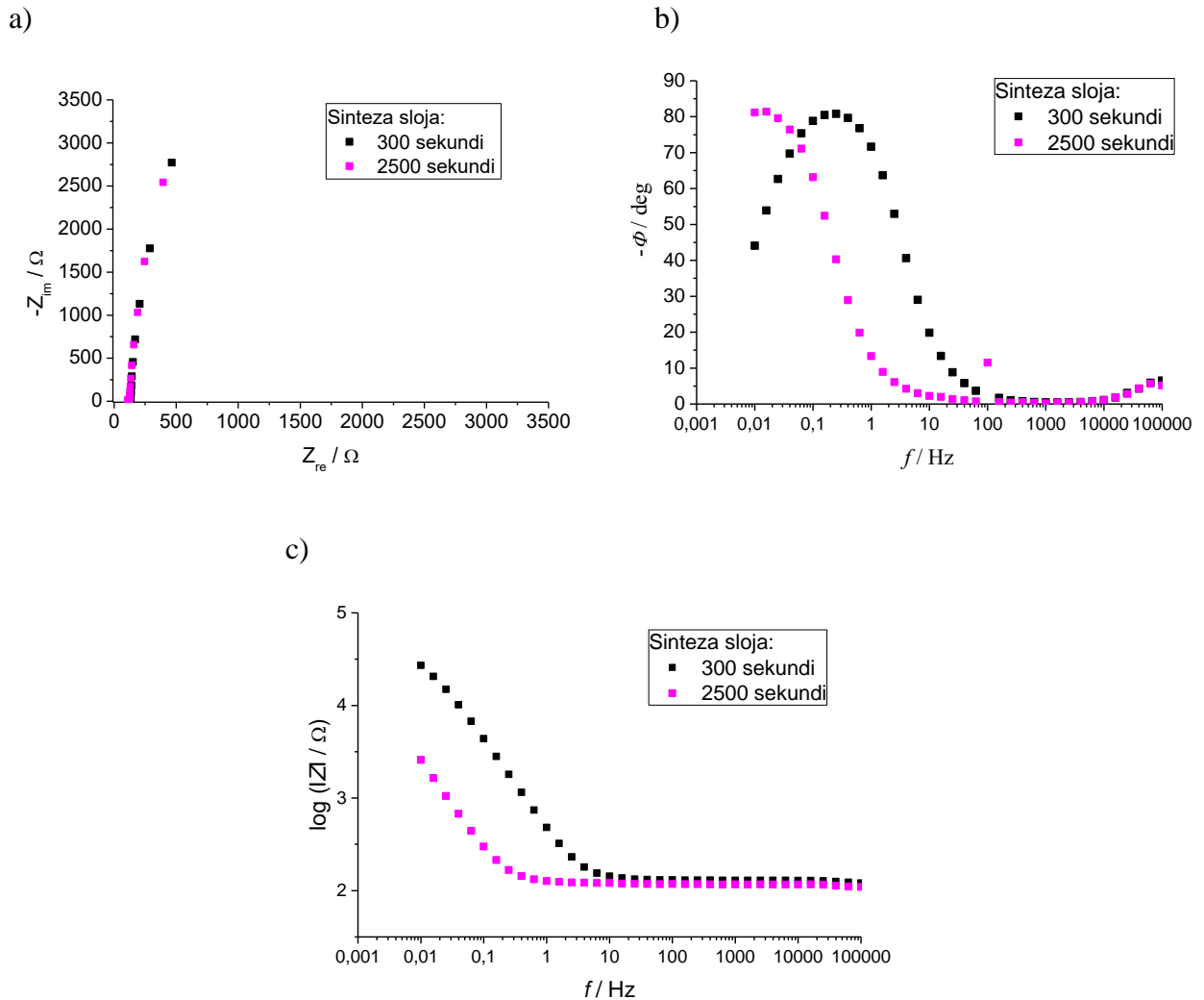
Slika 4.15. Odzivi zabilježeni metodom elektrokemijske impedancijske spektroskopije za različite PEDOT slojeve na potencijalu -0,3 V: a) Nyquistov prikaz, b) i c) Bodeov prikaz
