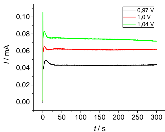
Slika 4.9. Strujni tranzijent zabilježen kod sinteze PEDOT/GO sloja u trajanju od 300 sekundi iz otopine 0,01 \text{ mol dm}^{-3} PSS, 2 \text{ mg mL}^{-1} GO i 0,02 \text{ mol dm}^{-3} EDOT pri različitim potencijalima
