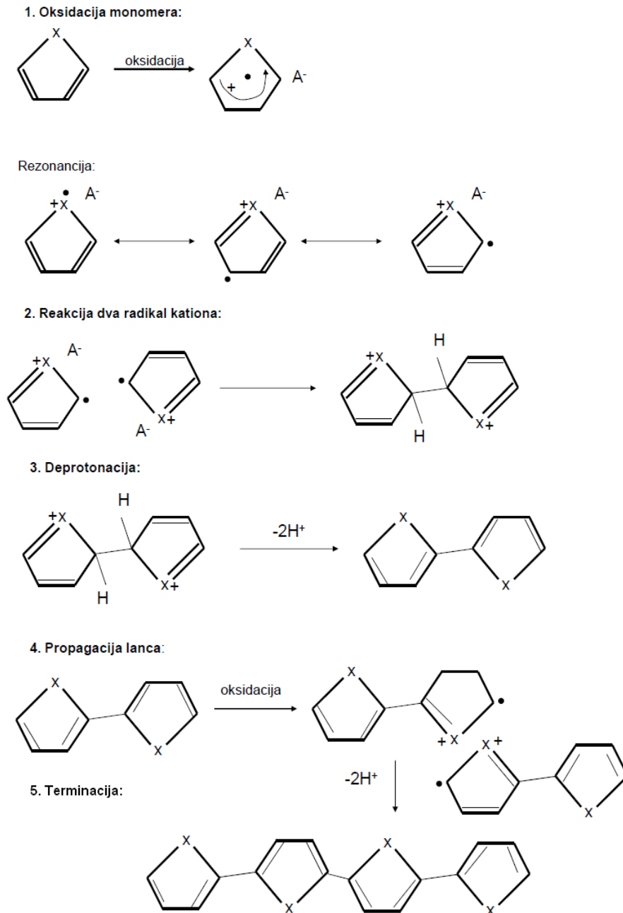
Slika 2.6. Shema polimerizacije
