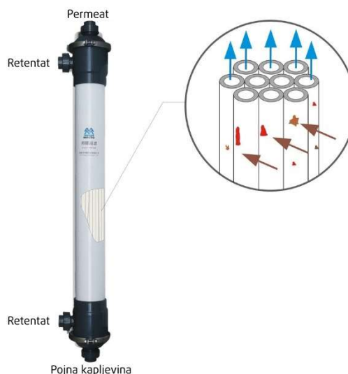
Slika 6. Membranski modul u obliku šupljih vlakana
