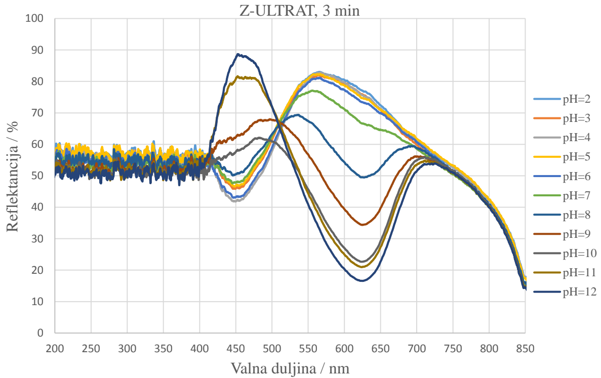
Slika 50. Spektrogram reflektancije filma BTf na materijalu Z-ULTRAT u smjeru rastećeg pH
