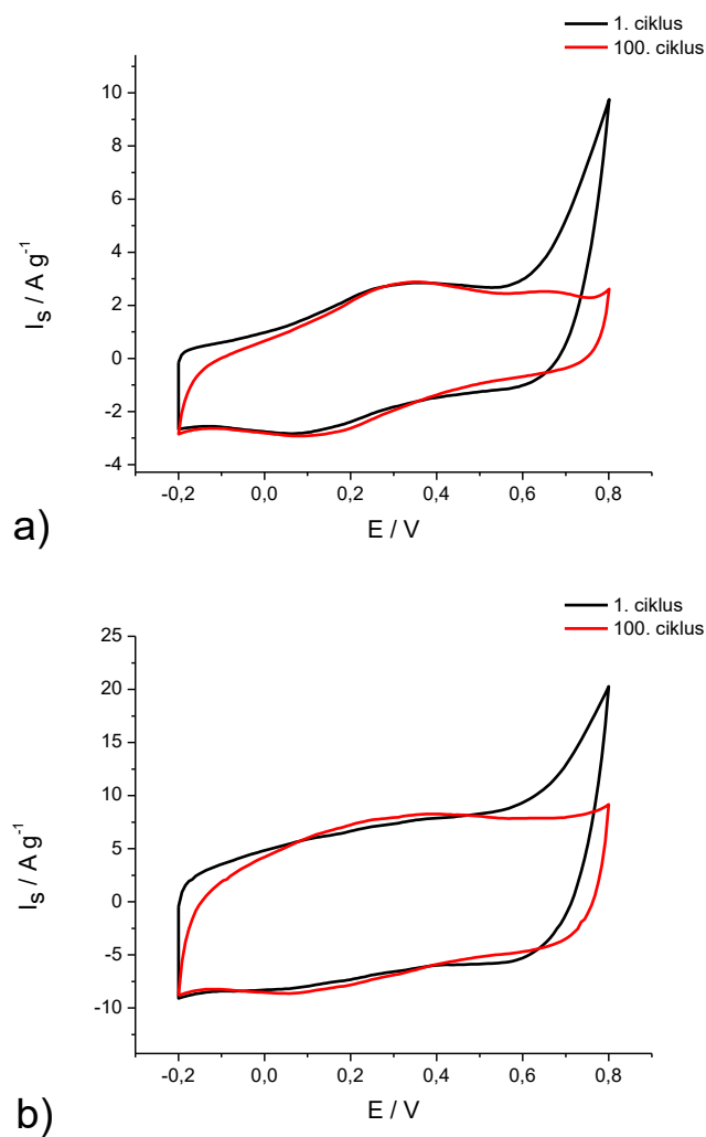
Slika 4.7 Ciklički voltamogrami elektroda a) rGO-PPy-0 i b) rGO-PPy-7 snimljeni u području potencijala od -0,2 V do 0,8 V, u elektrolitu \text{H}_2\text{SO}_4 .
