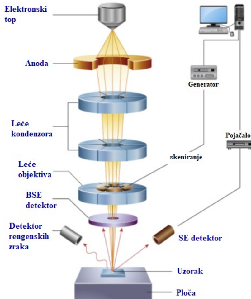
Slika 14. Shematski prikaz glavnih dijelova pretražnog elektronskog mikroskopa. Slika preuzeta i modificirana [66].
