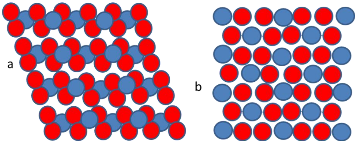
Slika 1. a) Shematski prikaz monoklinske strukture VO 2 (M) i b) rutilne strukture VO 2 (R)
