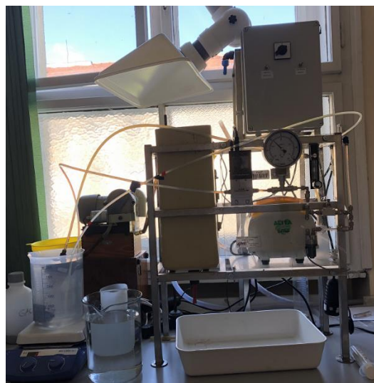
Slika 13. a) Shematski i b) slikovni prikaz laboratorijskog uređaja
