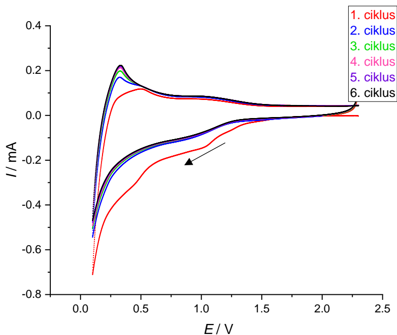
Slika. 4.1.1. Ciklička voltometrija za članak PSi4. Početni napon, E_p=2,3 V, konačni napon, E_k=0,1 V, brzina promjene napona, \nu=10 mV.
